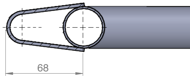
A-A (1 : 2)
