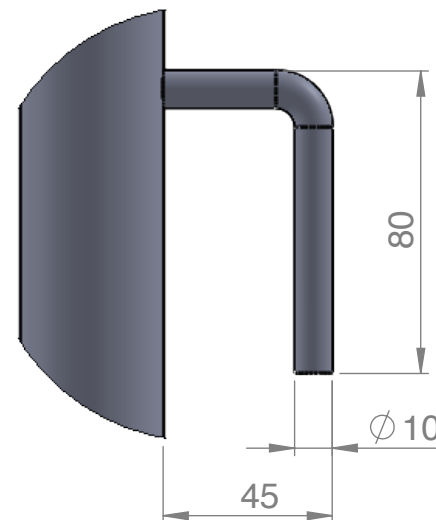
B (1 : 2)
